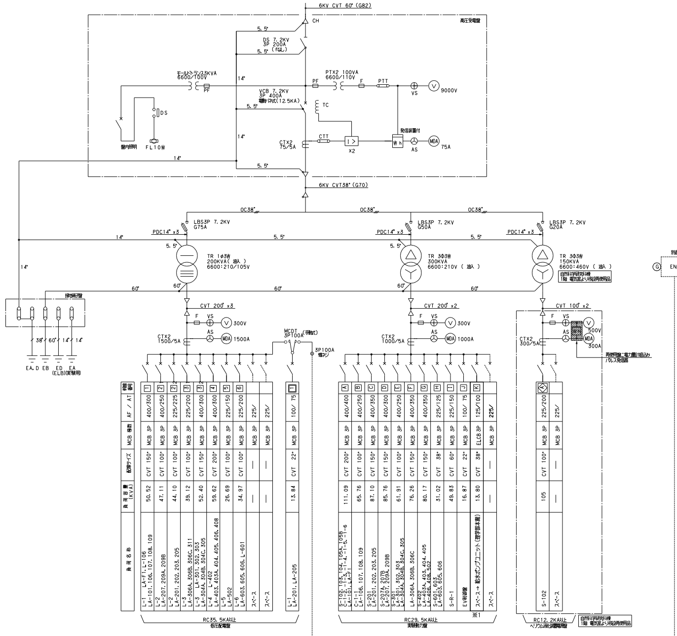
受変電設備 単線結線図
