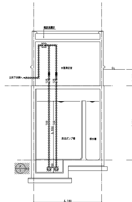
A-A' 断面図 S=1/50
