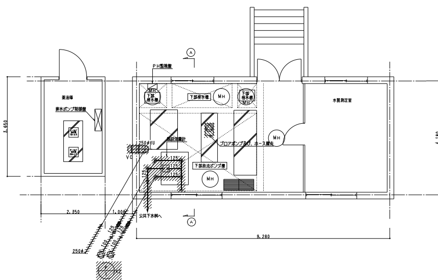
北団地下水質測定室 平面図 S=1/50
