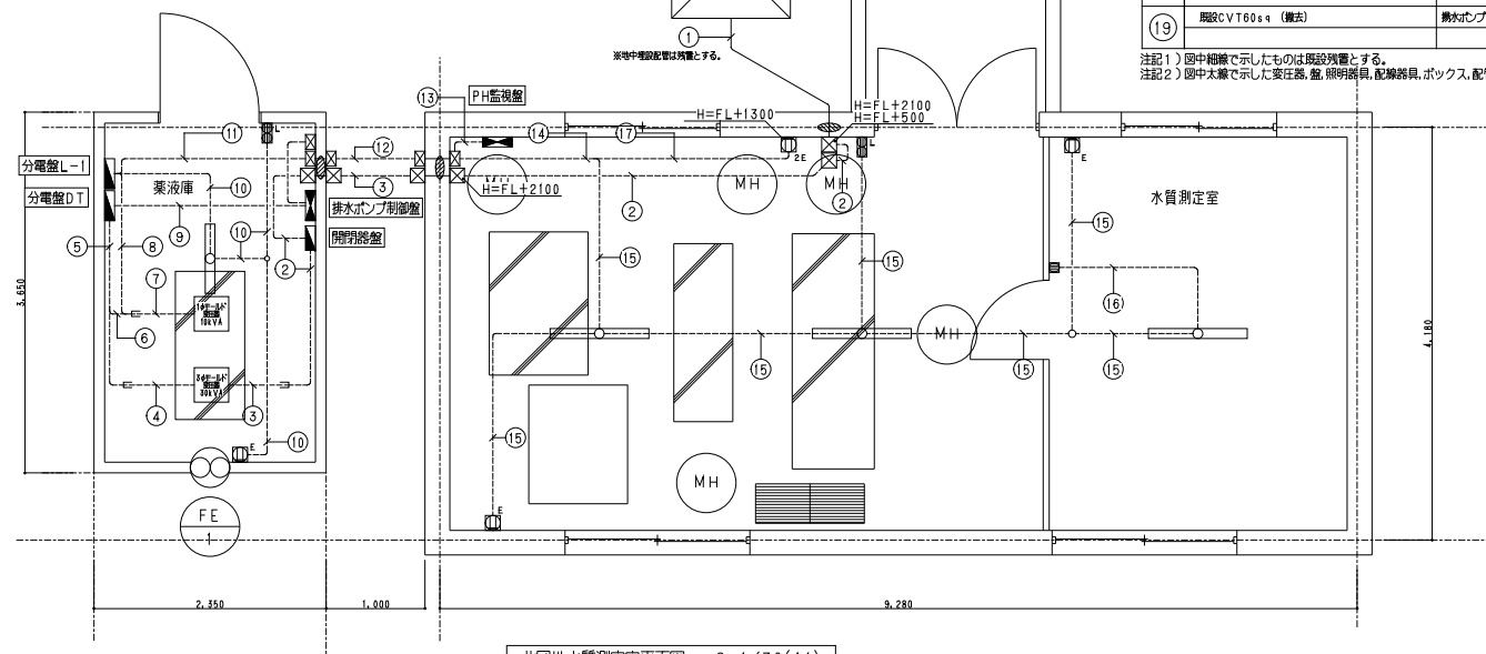
北団地水質測定室平面図 S=1/30(A1)
